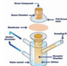
Gambar 1. Alat Sel Difusi Franz
